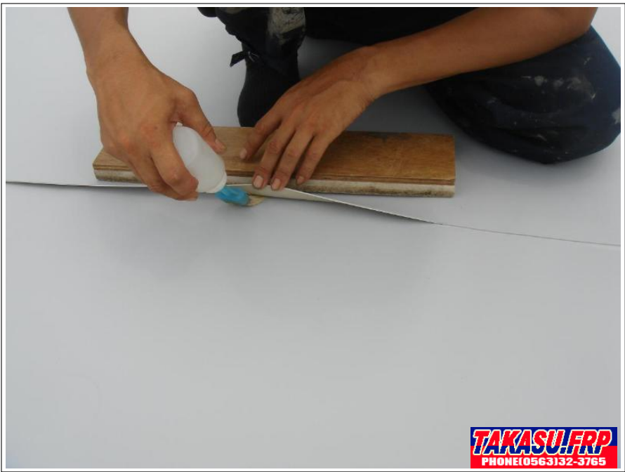
塩ビシートジョイント融着
